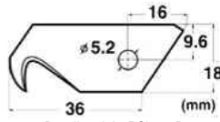
Detailansicht BSL-21P
