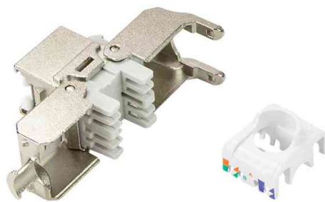
Keystone Modul Kat.6A, geschirmt
